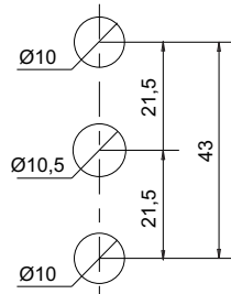
CAJEADO TRANSMISIÓN
